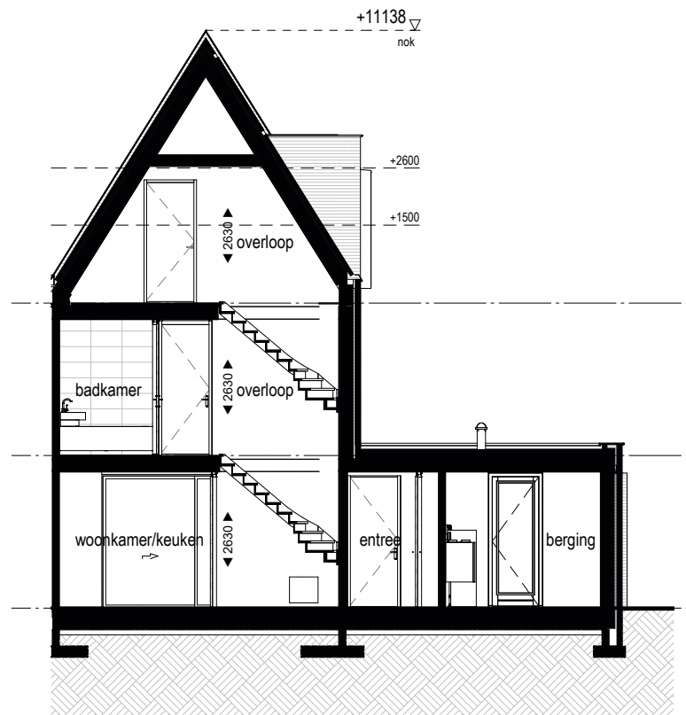
Doorsnede B
