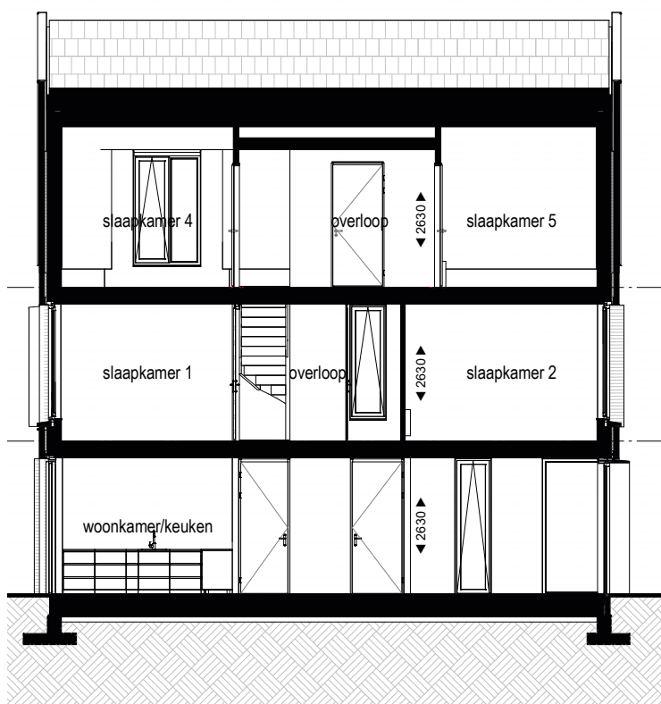
Doorsnede A
