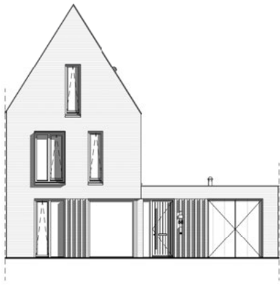
voorgevel
