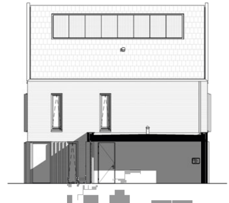
zijgevel
