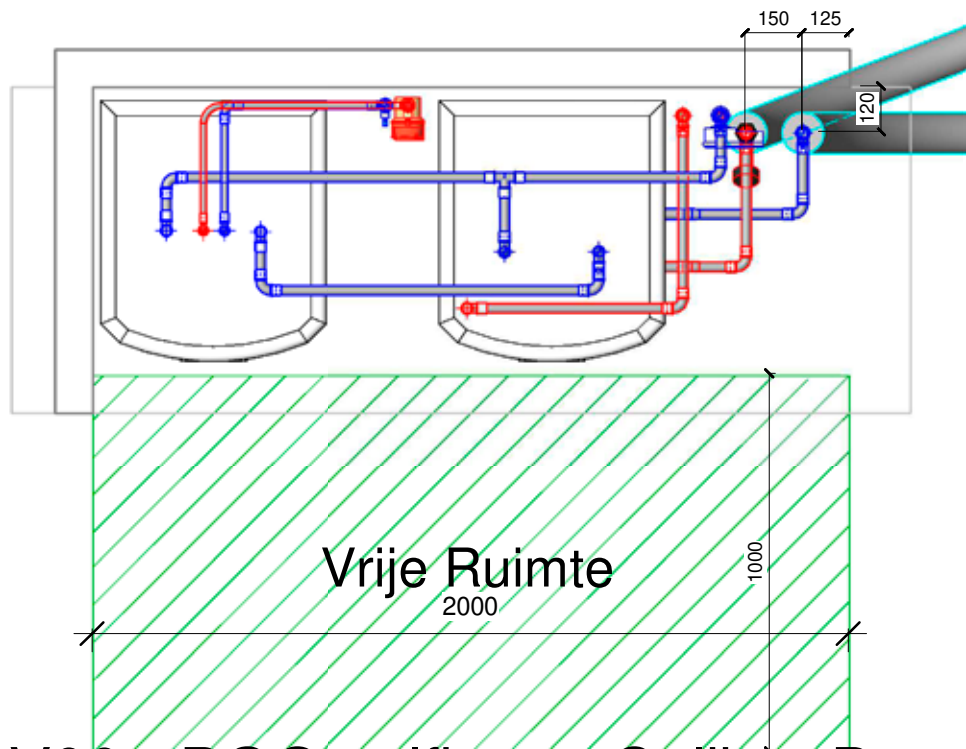
1 V00 - BGG zelfbouw Calibra Duo 1 : 20
